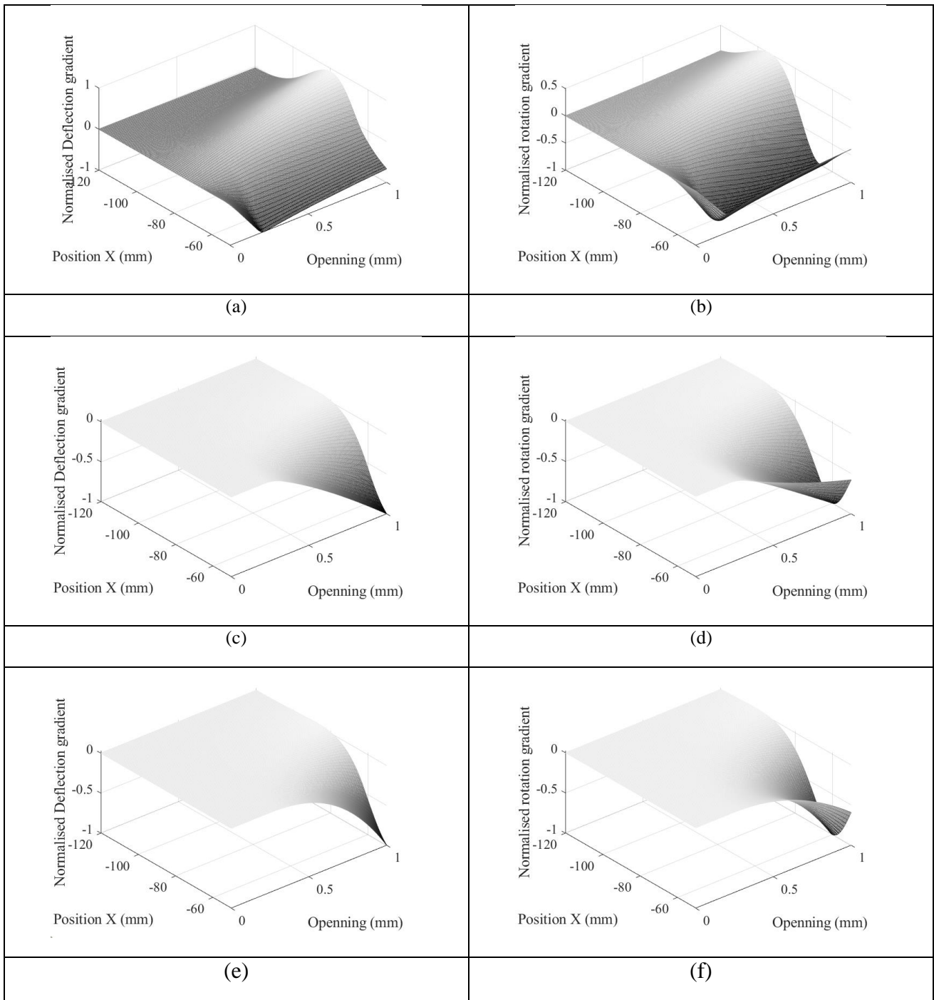
Figure 8 : Fonctions des sensibilités obtenue par CIN respectivement en déplacement et rotation : (a) et (b) Sensibilité au module ;(c) et (d) Sensibilité à la contrainte maximale ; (e) et (f) Sensibilité au taux de restitution d'énergie critique.
