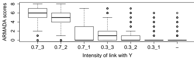
FIGURE 7 – Scénario 2 : moyennes et boxplots des scores calculés sur N = 100 runs de (\mathbf{X}, Y) .
