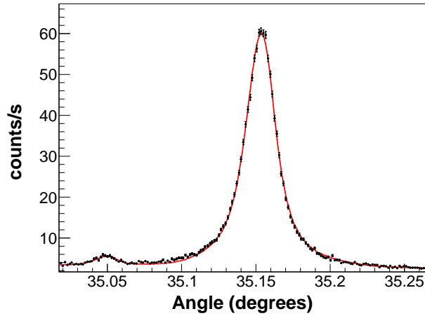
(a) 1s\ 2s\ 2p\ ^4P_{5/2} \rightarrow 1s^2\ 2s^2\ ^2S_{1/2} and 1s\ 2s^2\ 2p\ ^1P_1 \rightarrow 1s^2\ 2s^2\ ^1S_0 .
