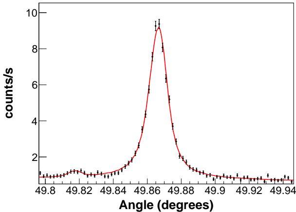
(a) 1s\ 2s\ 2p\ ^4P_{5/2} \rightarrow 1s^2\ 2s^2\ ^2S_{1/2} and 1s\ 2s^2\ 2p\ ^1P_1 \rightarrow 1s^2\ 2s^2\ ^1S_0 .
