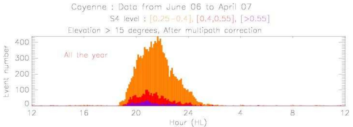
Figure 9. Histogramme des événements de scintillation à Cayenne pour la période de juin 2006 à juillet 2007. L'intensité des scintillations est évaluée à l'aide de l'indice S4 selon le code de couleurs : Scintillations fortes (mauve), moyennes (en rouge), faibles (ocre) [13].
