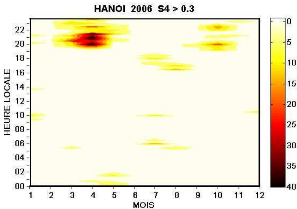
Figure 10. Histogramme des évènements de scintillation à Cayenne et à Hanoi en fonction du mois et de l'heure locale pour des scintillations correspondant à un indice S4 > 0,3 . Le code de couleurs représente le nombre d'évènements durant une tranche de temps de 15 minutes ; (a) station de Cayenne (Guyane française) de juin 2006 à juillet 2007 ; (b) station de Hanoi (Vietnam) pour l'année 2006.
