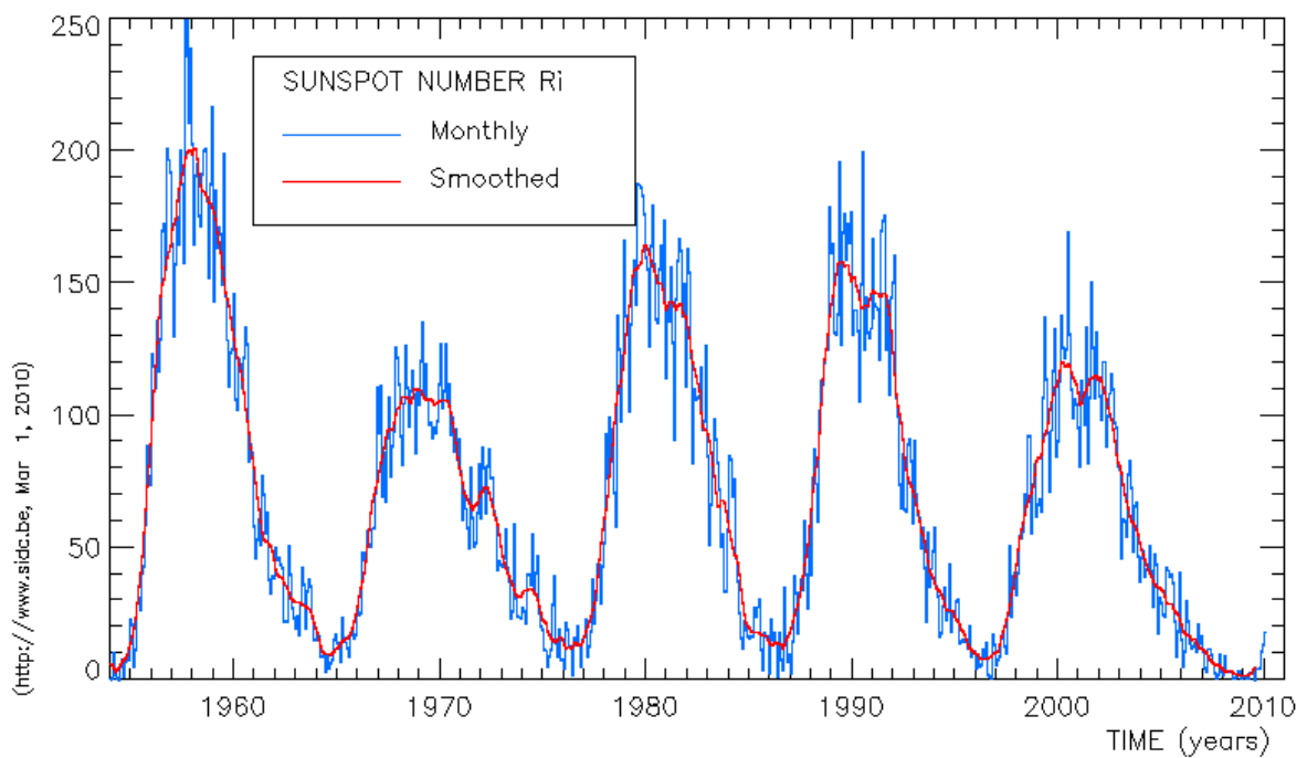
Figure 3 – Valeur de l'indice solaire depuis 1950 montrant les cinq derniers cycles d'activité solaire [7].
