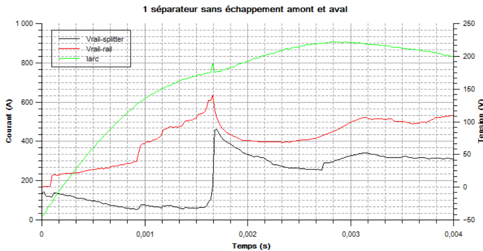
Fig. 2. Résultat expérimental avec 1 séparateur sans échappement en amont et aval
