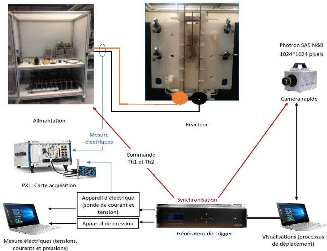
Fig. 1. Dispositif expérimental utilisé pour les tests
