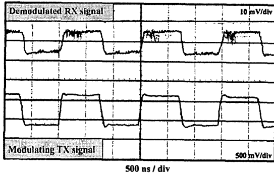
b) Module 1 = Modulator
