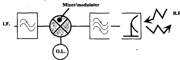
Fig. 3. Dual mode RX/TX module : schematic
