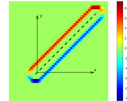
(d) \frac{\partial \delta}{\partial Y} , R = dx , N_{gp} = 4
