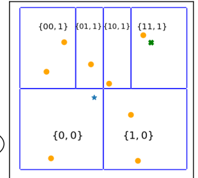
Cellule de l'arbre iSAX - 2D
