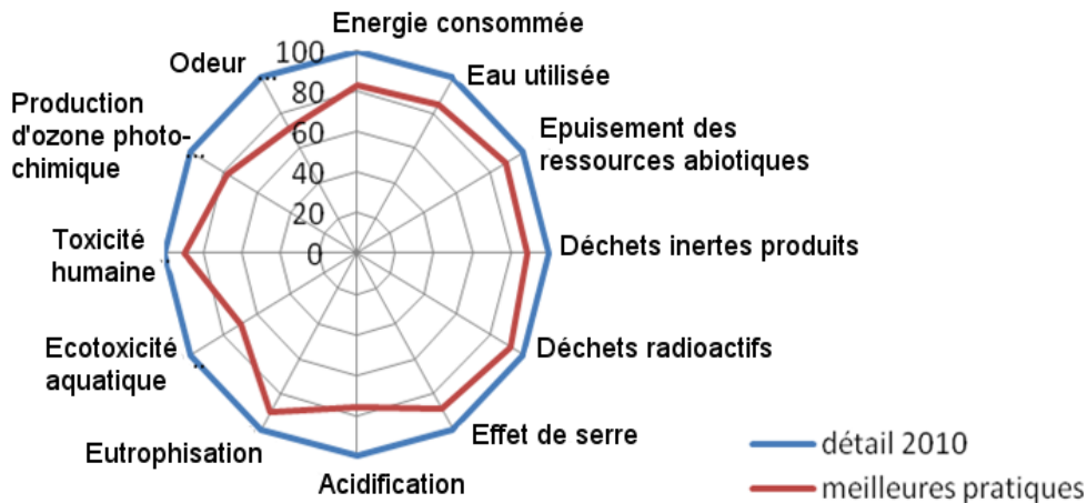
Figure 8. Analyse de cycle de vie comparative des deux variantes pour le plan de masse 2010 (logiciel ARIADNE)
