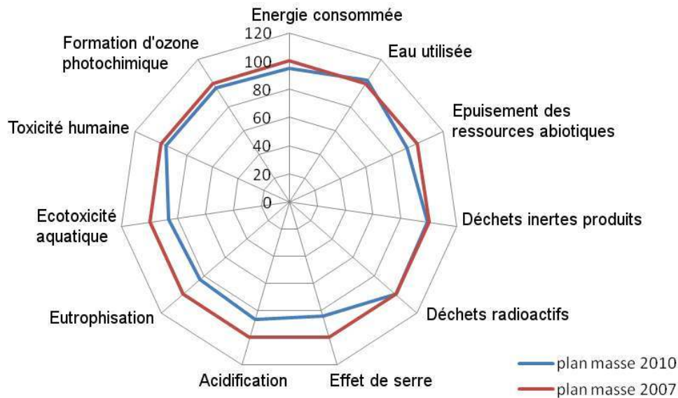
Figure 7. Analyse de cycle de vie comparative des plans de masse de 2007 et 2010 (logiciel ARIADNE)
