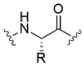
\alpha -peptides
