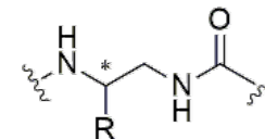
oligoureas
