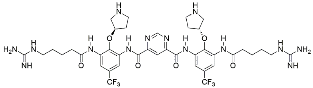
Brilacidin (58)
