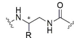
oligoureas
