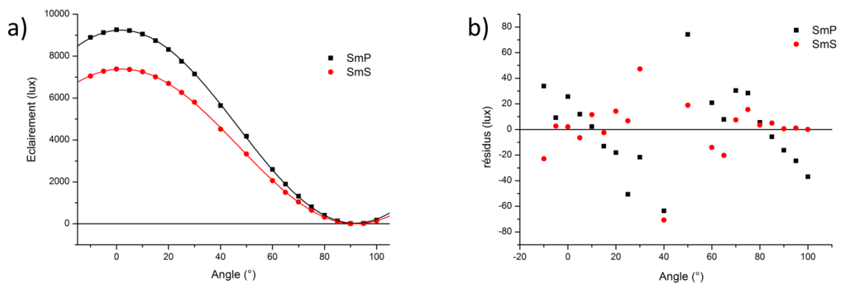
Figure 4 : a) Éclairages transmis en fonction de l'angle entre polariseur et analyseur et ajustements. b) Résidus apparemment aléatoires sauf peut-être les mesures à 40° et 50° pour lesquelles les résidus semblent être légèrement excessifs.
