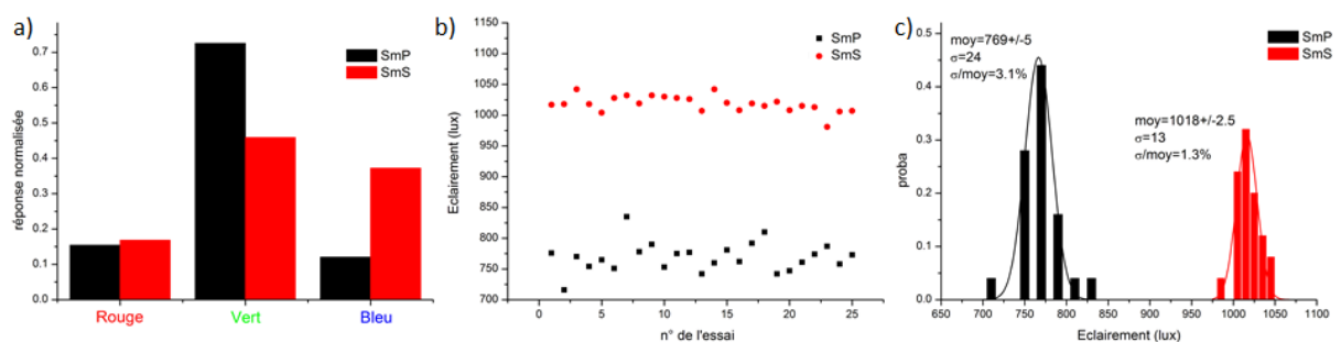
Figure 3 : a) Sensibilité spectrale relative des deux smartphones. b) répétabilité de la mesure de la transmission à travers un seul transparent. c) statistiques pour les 25 répétitions de la mesure.
