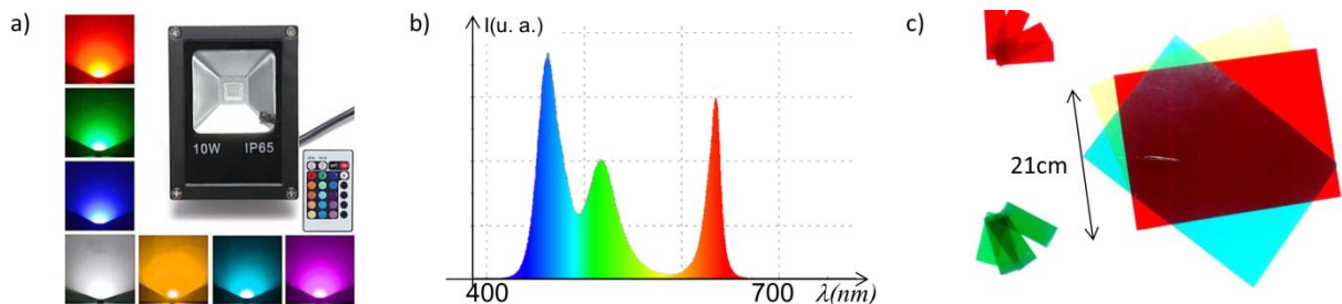
Figure 2 : a) projecteur utilisé et sa télécommande. b) spectre d'émission des trois jeux de LEDs. Rouge : 630 \pm 8 nm, vert : 514 \pm 14 nm, bleu : 448 \text{ nm} \pm 10 \text{ nm} . c) transparents colorés : à droite sous forme de feuilles A4, à gauche les échantillons rouges et verts utilisés.
