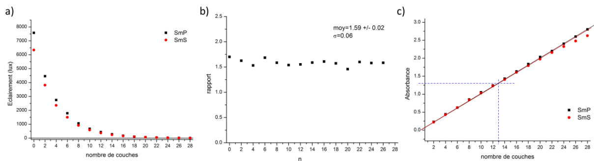
Figure 5 : a) Eclairement transmis en fonction du nombre de couches. b) rapport des éclairements pour n et n+2 couches. c) Absorbance en fonction du nombre de couches et ajustements linéaires. Pour SmS on note une légère déviation aux fortes absorbances. Seuls les 11 premiers points sont pris en compte pour l'ajustement. Les pointillés bleus correspondent à la détermination du nombre de couches d'un échantillon inconnu (voir IV1c).
