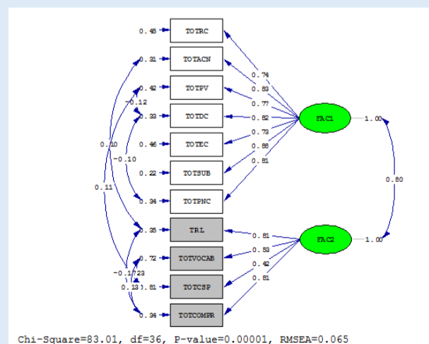
Figure 1 : Analyse factorielle confirmatoire de l'ensemble des épreuves (modèle à deux facteurs)
