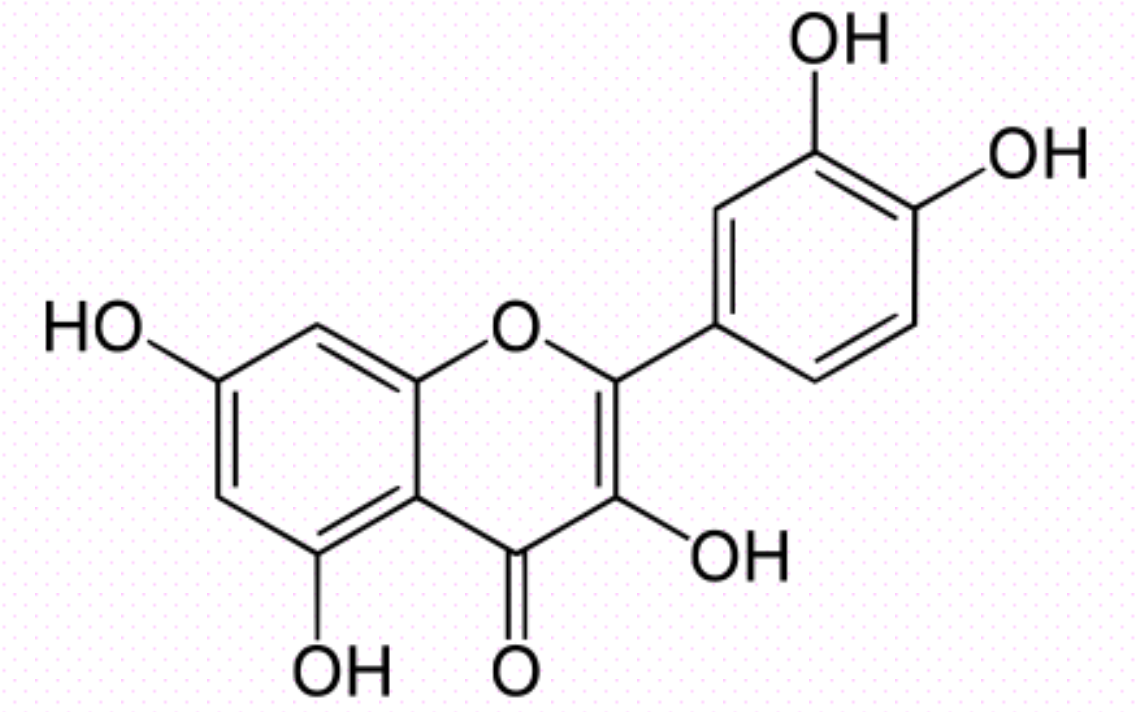
Slika 1. Struktura kvercetina
