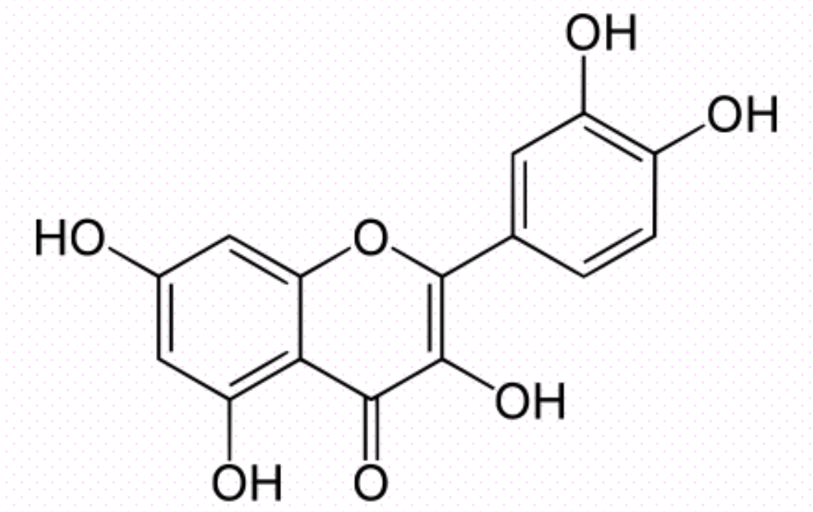
Slika 1. Struktura kvercetina
