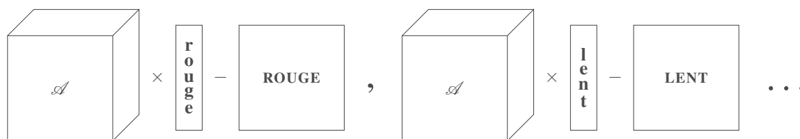
FIGURE 4: Apprentissage du tenseur \mathcal{A}
