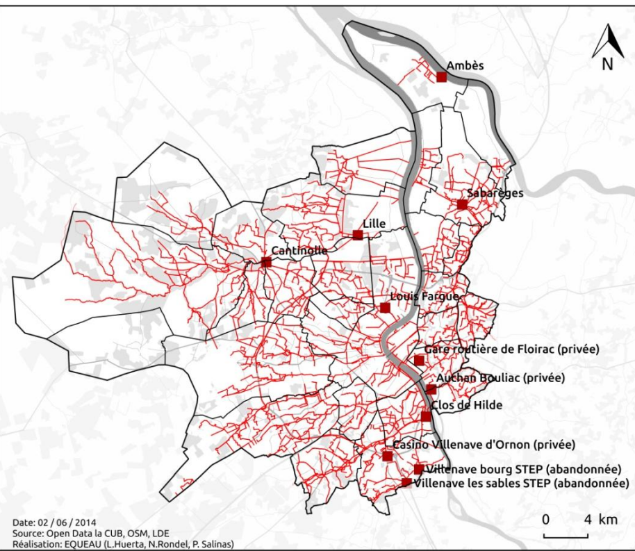
Le réseau d'assainissement de la CUB
