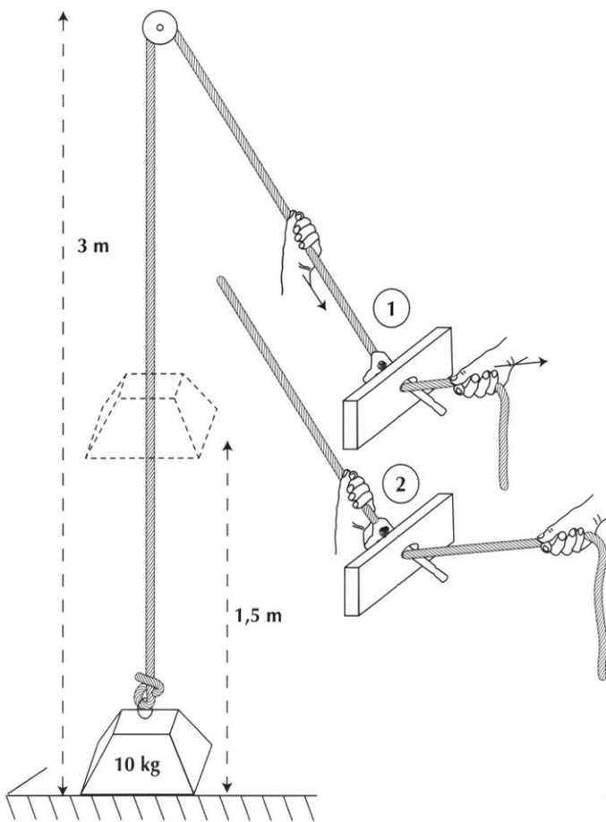
Fig. 4 – Paramètres expérimentaux constants : 1, traction des deux mains à la fois ; 2, quand la main gauche arrive au contact du bâton percé, coinçage de la corde et retour à la position 1.
