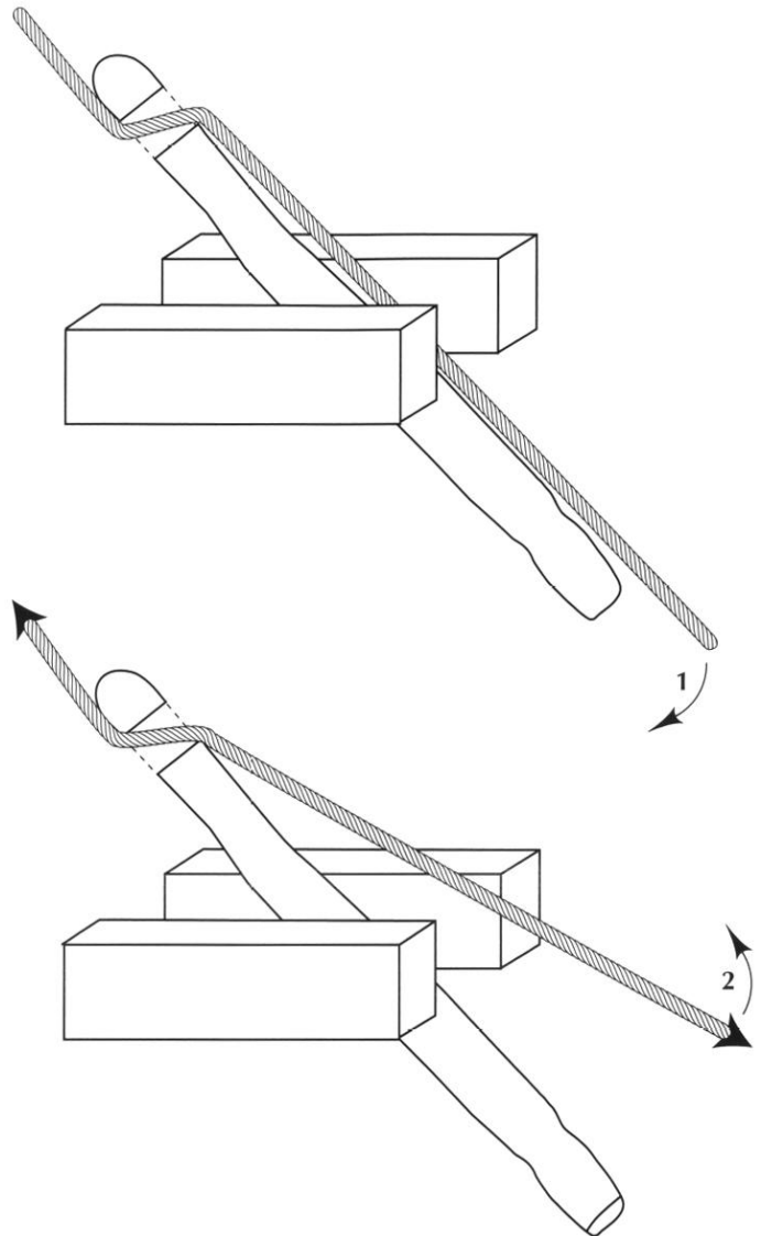
Fig. 11 – Expérience 3. Bâton n° 2 fixé directement dans l'étau : 1, en plaquant la corde sur le fût toute circulation devient impossible ; 2, en éloignant la corde du fût, elle peut circuler dans les deux sens.
