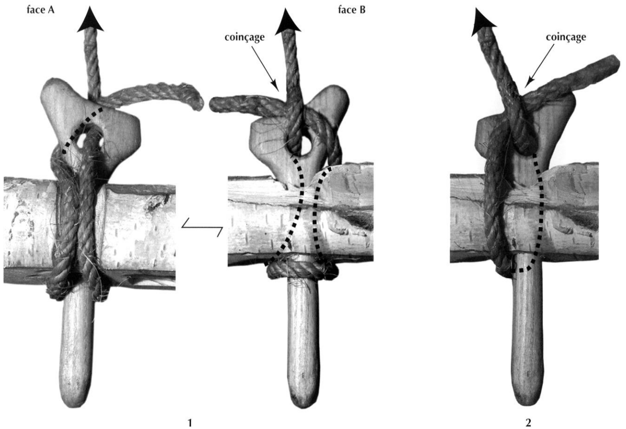
Fig. 14 – Expérience 4 (bâton n° 3) : deux possibilités de coinçage rapide de la corde sans utiliser un nœud. La flèche indique le sens de la traction exercée par le poids.
