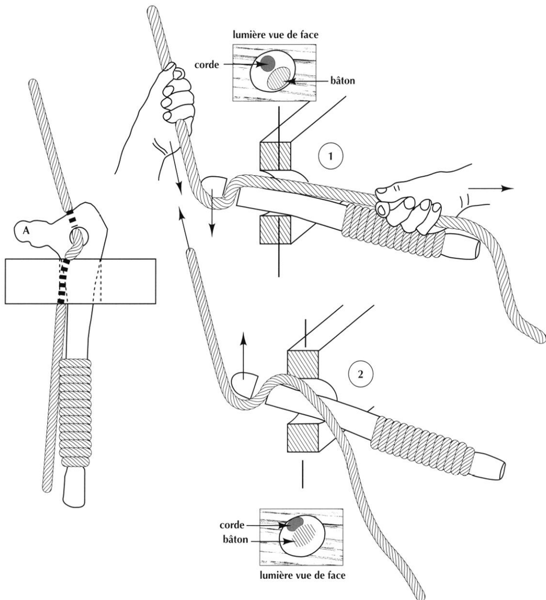
Fig. 6 – Expérience 1 (bâton n° 1). Halage du poids : 1, la traction de la main gauche sur la corde soulage le bâton qui libère le passage en haut de la lumière. Simultanément, la main droite fait glisser la corde à travers le bâton et la lumière ; 2, quand la traction de la main gauche cesse, le poids tire sur la corde, le bâton remonte et coince la corde contre le bord supérieur de la lumière.
