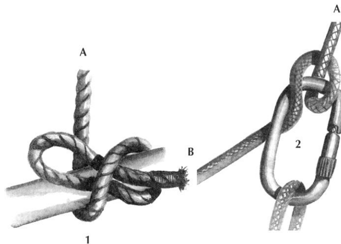
Fig. 15 – 1, nœud de drisse : une traction sur le brin B libère le brin A ; 2, nœud de Munter utilisé en escalade : tant qu'une tension s'exerce sur le brin B, le brin A ne peut pas coulisser (d'après F. Ripault).
