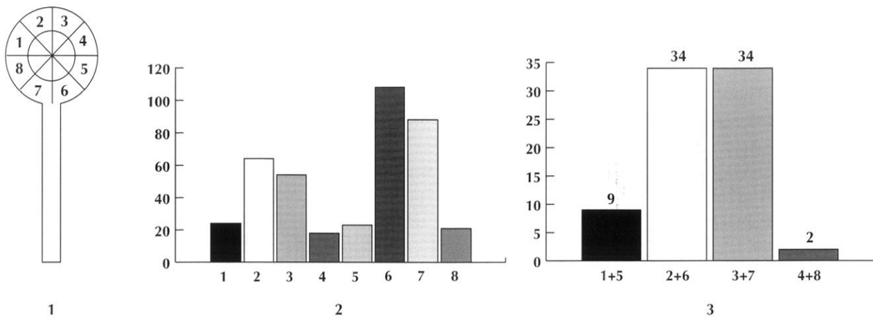
Fig. 2 – 1, cadran Glory définissant les zones d'usure de l'œil ; 2, répartition des usures constatées par Glory sur 115 bâtons percés pour chaque secteur ; 3, total des usures alternes diamétralement opposées.
