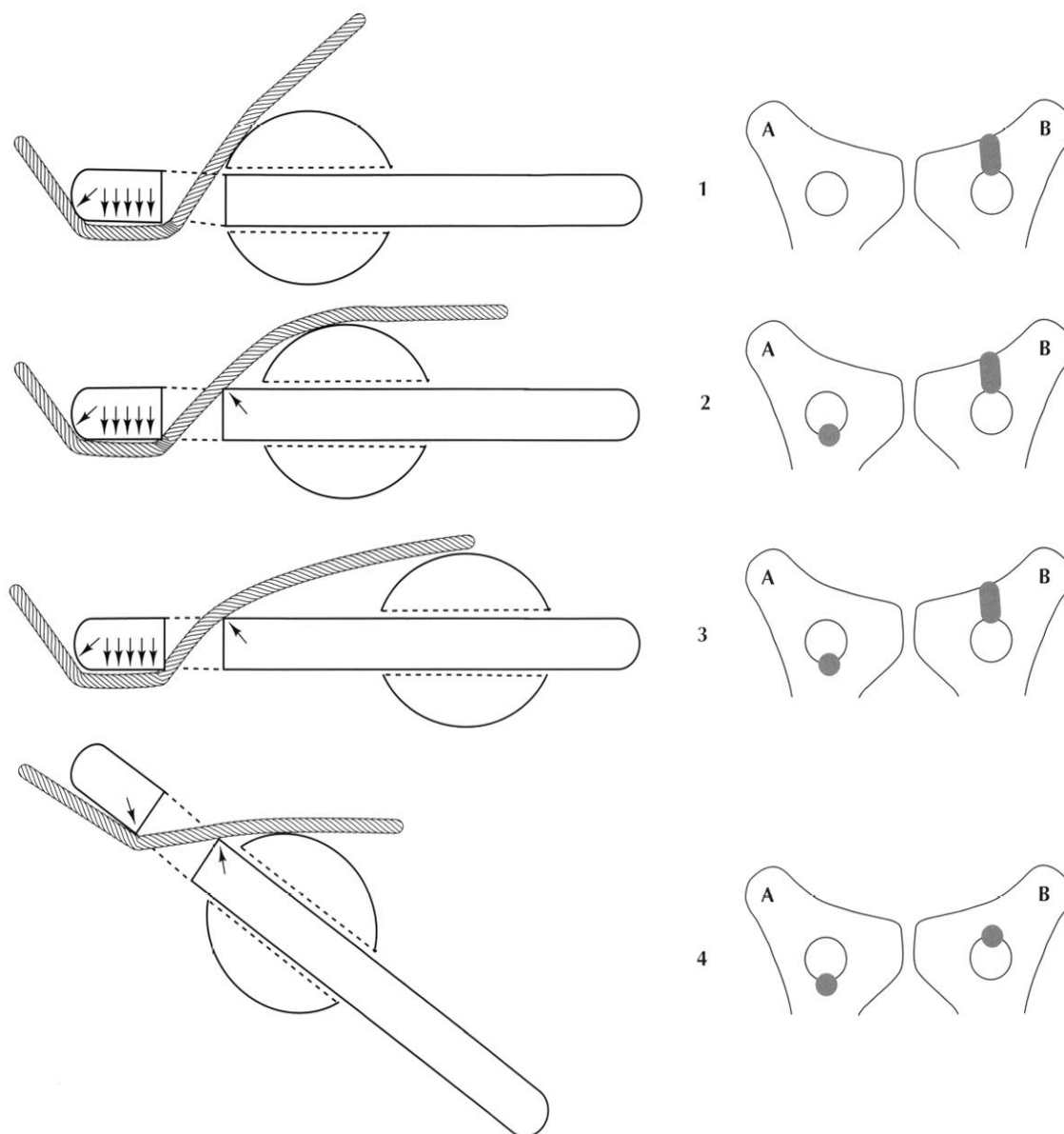
Fig. 16 – Expérience 4. Variation de la place et de l'étendue des usures sur le bâton n° 3 : 1-3, en fonction de la position du bâton par rapport au support ; 4, en fonction de l'inclinaison du bâton par rapport à l'horizontale.
