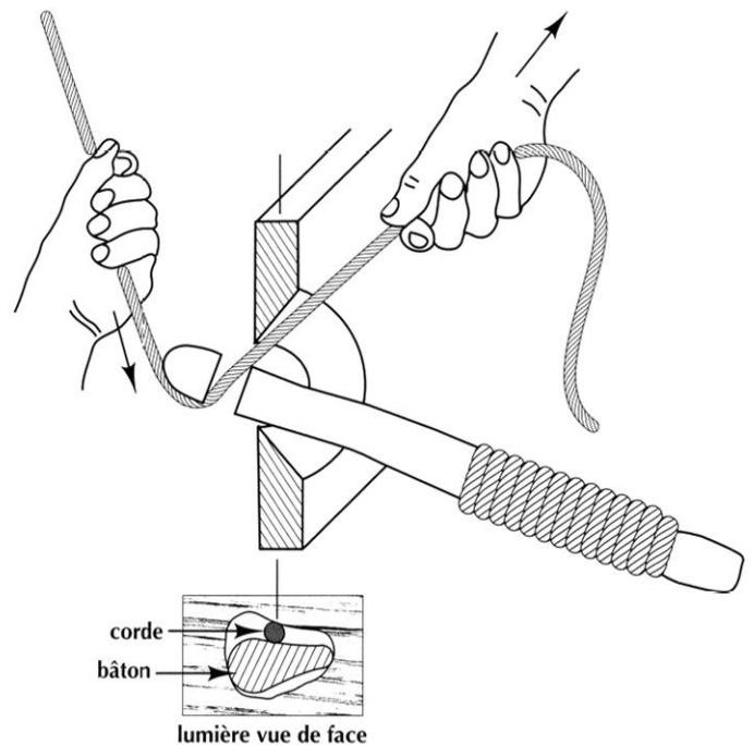
Fig. 9 – Expérience 2 (bâton n° 1). La lumière a été évasée vers l'arrière pour diminuer la friction de la corde sur le fût.
