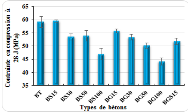
Figure 1. Evaluation des résistances caractéristiques des différents bétons
