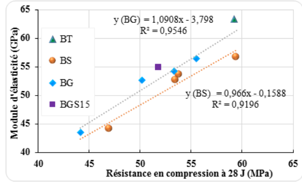
Figure 2. Relations entre le module d'élasticité et la résistance caractéristique des différents bétons
