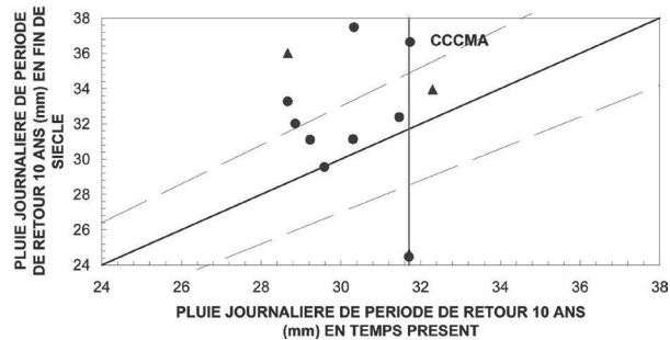
Figure 4 : Évolution des quantiles décennaux de la précipitation moyenne à l'amont de Paris entre le climat présent (PST) et la fin du siècle (FS) : maximum journalier annuel PJXA10 et maximum annuel du cumul sur 12 jours P12JXA(T = 10 \text{ ans}) . Un point par scénario climatique régionalisé (● : scénarios régionalisés A1B ; ▲ : scénarios régionalisés A2 – issus du modèle climatique ARPEGE). La droite oblique est la première bissectrice et celles en tireté définissent les enveloppes à \pm 10 \% des valeurs PST. La droite verticale rouge donne les quantiles décennaux déduits des précipitations SAFRAN pour la période PST.
