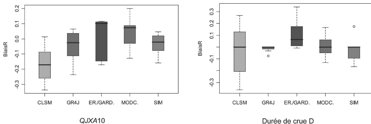
Figure 2 : Écart relatif médian entre les valeurs temps présent et milieu de siècle des variables retenues pour caractériser des crues dans l'ensemble des stations du domaine RExHySS (Seine et Somme).
