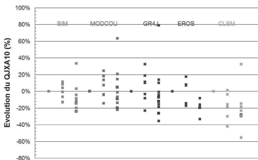
Figure 3 : Évolution du QJXA10 simulé pour la Seine à Paris. Les évolutions sont calculées par rapport aux débits simulés sous scénarios désagrégés temps présent. Pour chaque scénario, la première valeur correspond aux résultats temps présent (0 % de changement relatif quel que soit le scénario), la deuxième (lorsqu'elle existe) au milieu de siècle, et la troisième à la fin de siècle. Les points entourés en noir correspondent aux scénarios A2.
