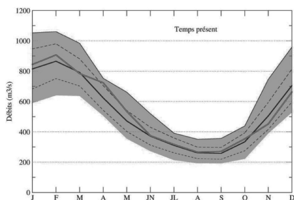
Figure 1 : Évolution des débits mensuels simulés pour la Seine à Poses par l'ensemble des modèles hydrologiques et sur l'ensemble des scénarios. L'enveloppe représente les min et max simulés, le trait épais noir la moyenne de l'ensemble, et les pointillés l'enveloppe pour un écart-type. Temps présent : la courbe rouge représente la moyenne mensuelle observée. Horizon 2050 : la courbe bleue représente la moyenne temps présent. Horizon 2100 : les courbes bleues et roses représentent les moyennes des simulations temps présent et milieu de siècle respectivement.
