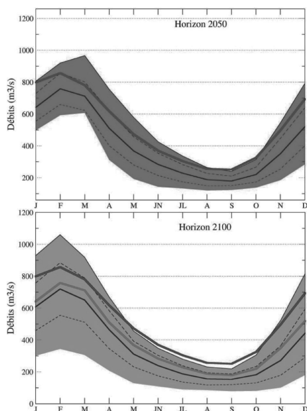
Figure 1 : Évolution des débits mensuels simulés pour la Seine à Poses par l'ensemble des modèles hydrologiques et sur l'ensemble des scénarios. L'enveloppe représente les min et max simulés, le trait épais noir la moyenne de l'ensemble, et les pointillés l'enveloppe pour un écart-type. Temps présent : la courbe rouge représente la moyenne mensuelle observée. Horizon 2050 : la courbe bleue représente la moyenne temps présent. Horizon 2100 : les courbes bleues et roses représentent les moyennes des simulations temps présent et milieu de siècle respectivement.
