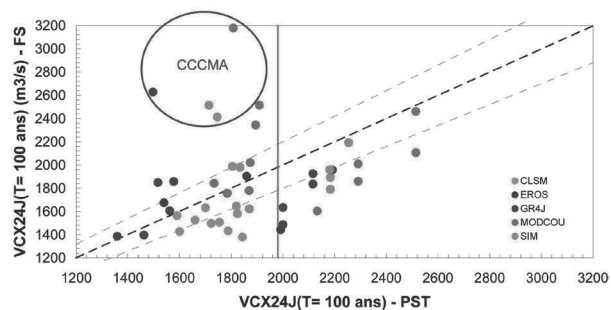
Figure 5 : Évolution des quantiles centennaux du débit à Paris entre le climat présent (PST) et la fin du siècle (FS) : débits moyens sur 24 jours VCX24J(T = 100 \text{ ans}) et débits journaliers QJXA100 . Un point par scénario hydrologique. La droite en tireté est la première bissectrice et celles en pointillé définissent les enveloppes à \pm 10 \% des valeurs PST. La droite verticale rouge donne les quantiles centennaux déduits des observations de débit [14].
