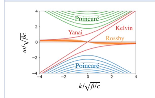
FIGURE 4 – Relation de dispersion sur le plan beta. On remarque trois différences avec le spectre des ondes peu profondes sur le plan f tracé figure 3 : (i) le spectre est discret (ii) la dégénérescence des modes géostrophiques est en partie levée, avec l'apparition des ondes de Rossby (orange) (iii) il existe deux nouveaux modes qui transitent d'une bande à l'autre : l'onde de Kelvin et l'onde de Yanai.
