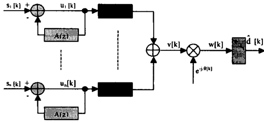
Fig. 2. SOC-MI-DFE (convergence mode).
