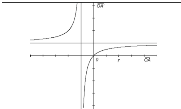
Figure.1 : Relation de conjugaison pour une lentille mince convergente. OA (resp. OA' ) abscisse du point de l'objet (resp. de l'image) situé sur l'axe optique. Pour une lentille mince divergente, la courbe s'obtient par symétrie de celle-ci par rapport à la première bissectrice. Pour les miroirs sphériques convexe et concave, ce sont les symétriques par rapport à l'un des axes des courbes associées aux lentilles (resp. convergente et divergente) qui interviennent.
