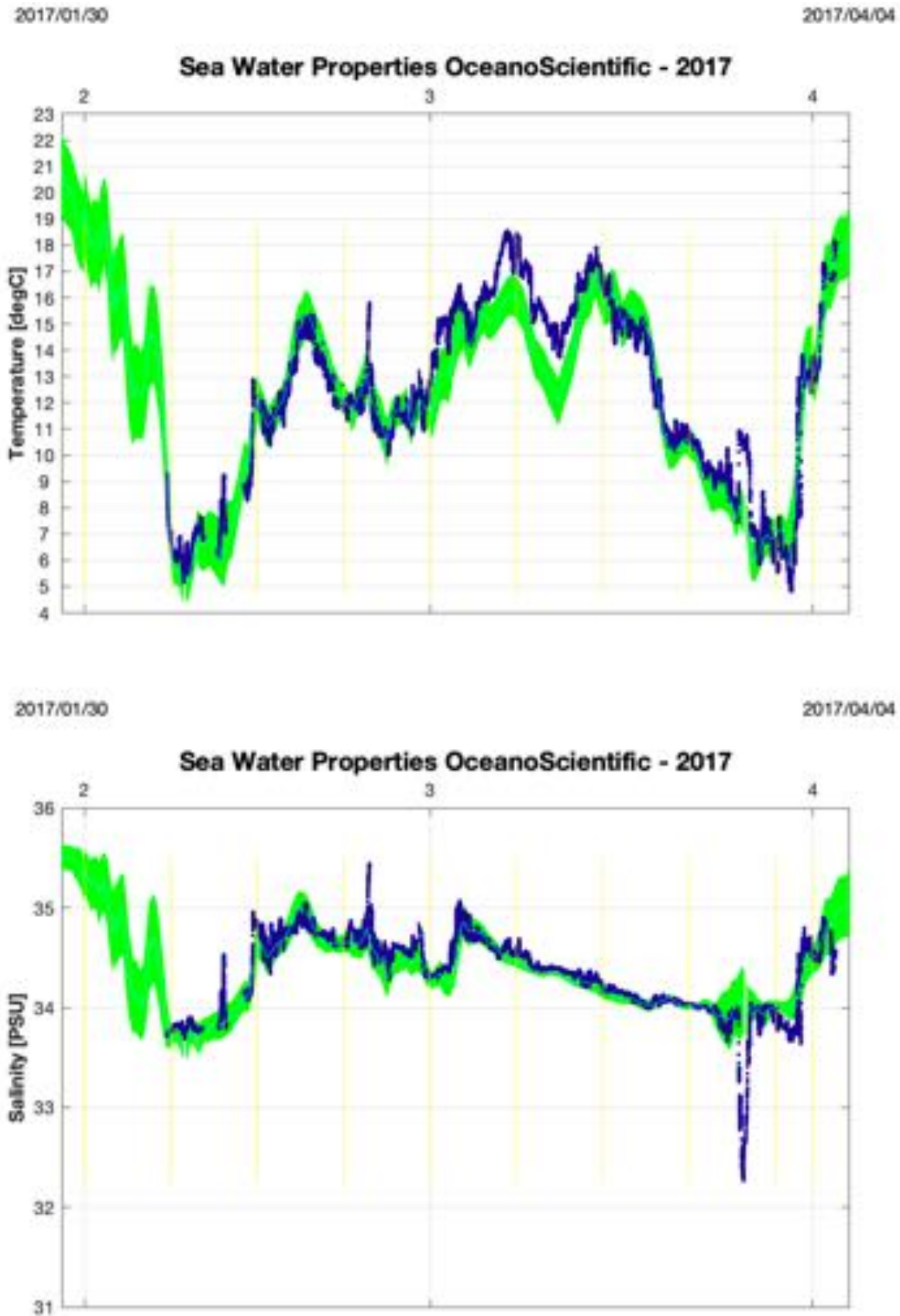
Figure 12 : Données de température et de salinité de l'Expédition OceanoScientific 2016-2017
