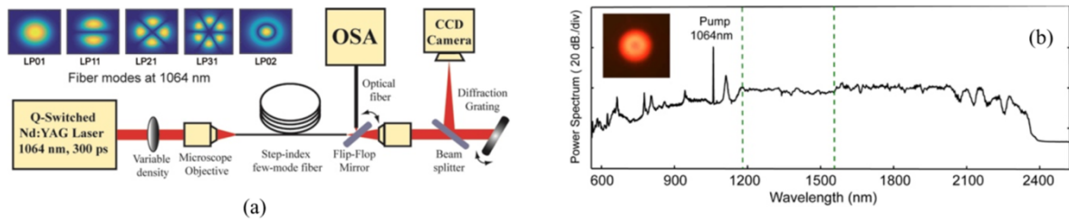
Figure 1 : (a) montage expérimental et (b) spectre du SC (560 nm \rightarrow 2350 nm) généré dans la fibre à saut d'indice de 50 m de long, mesuré avec 3 spectromètres optiques différents (les lignes en pointillés indiquent les 3 gammes de mesure utilisées). Puissance de sortie moyenne : 13 mW.
