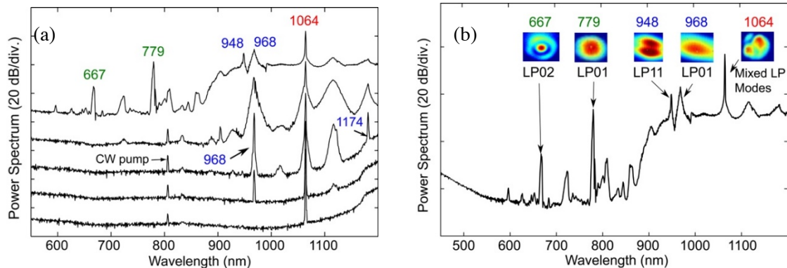
Figure 2 : (a) Spectres expérimentaux pour des puissances pompe de 0,85 mW, 1,6 mW, 2,6 mW, 3,5 mW et 8,1 mW (longueur de fibre : 5 m) ; (b) Spectre de sortie pour la puissance moyenne maximale. Les longueurs d'onde des composantes spectrales générées par FWM et les images des modes LP associés sont représentés.
