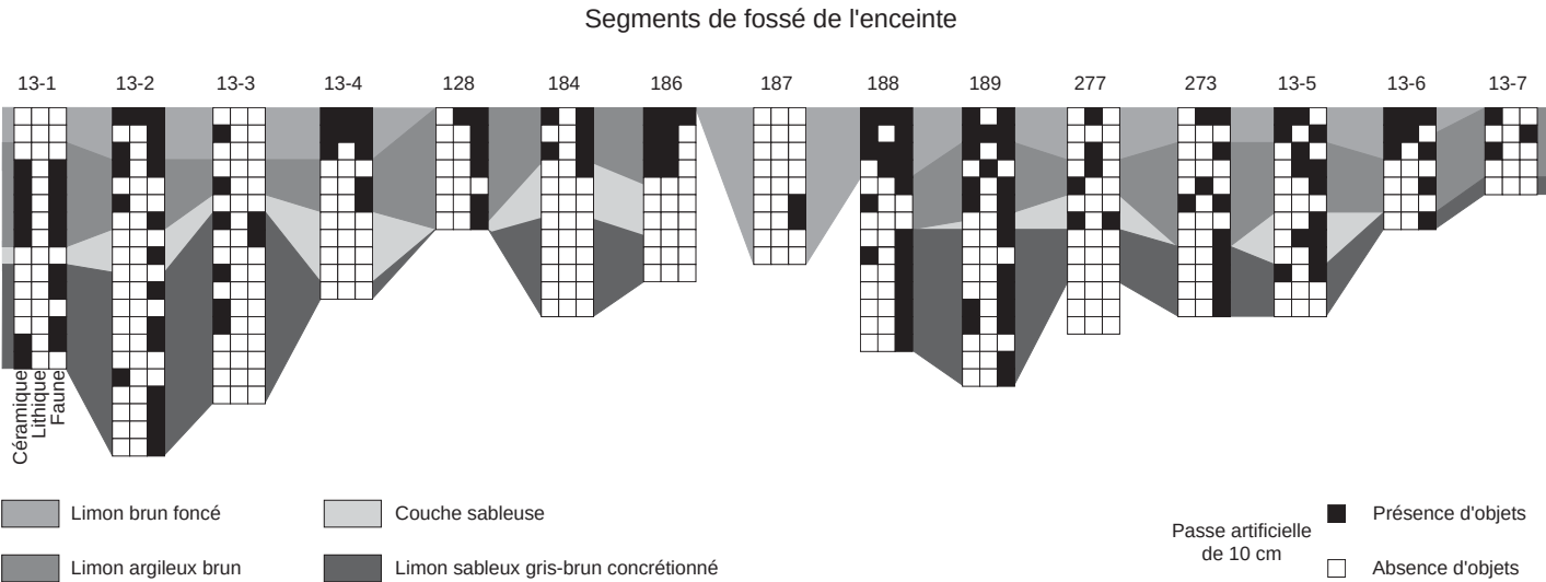
Fig. 5 – Stratigraphie schématique et distribution des trois principales catégories de vestiges (d'après Farruggia et al., 1996, fig. 34b ; DAO : C. Thevenet). Diagram of the stratigraphic sequence and distribution of the three main categories of remains (after Farruggia et al., 1996, fig. 34b; graphics: C. Thevenet).
