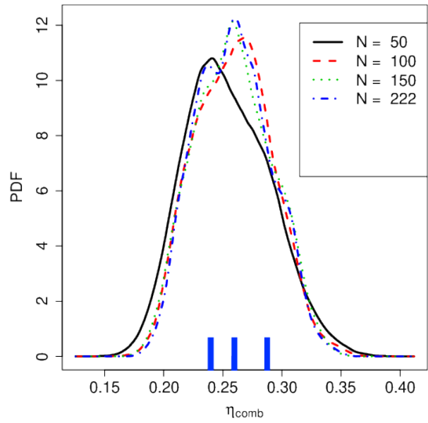
(d) Combustion efficiency, d/16 , \eta_{\text{comb}}
