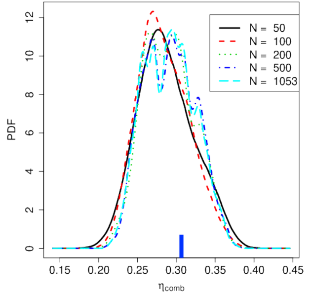
(d) Combustion efficiency, d/8 , \eta_{\text{comb}}
