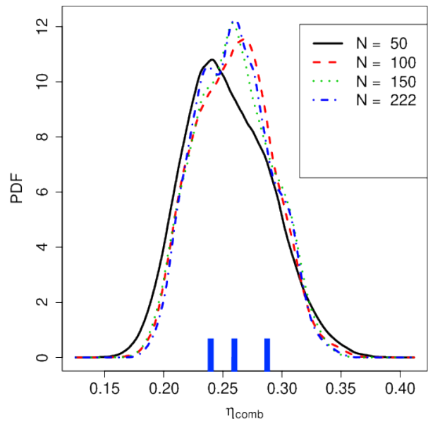
(d) Combustion efficiency, d/16 , \eta_{comb}
