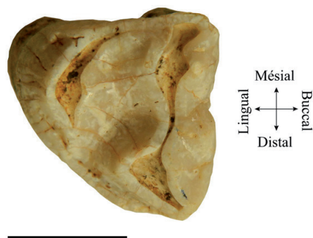
Fig. 8: Vue occlusale de la M2 gauche BEL XXIIS 1'12, Megaladapis sp. Echelle = 1 cm.
