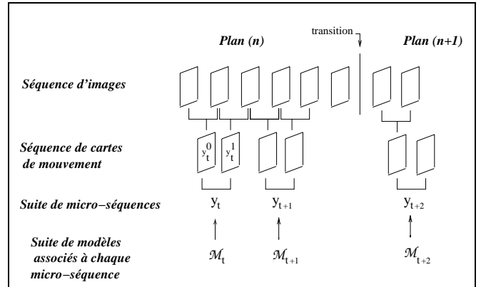
FIG. 1 – Décomposition de la séquence vidéo en micro-séquences de longueur 2 et modélisation statistique de l'activité de mouvement dans chacune d'entre elles.
