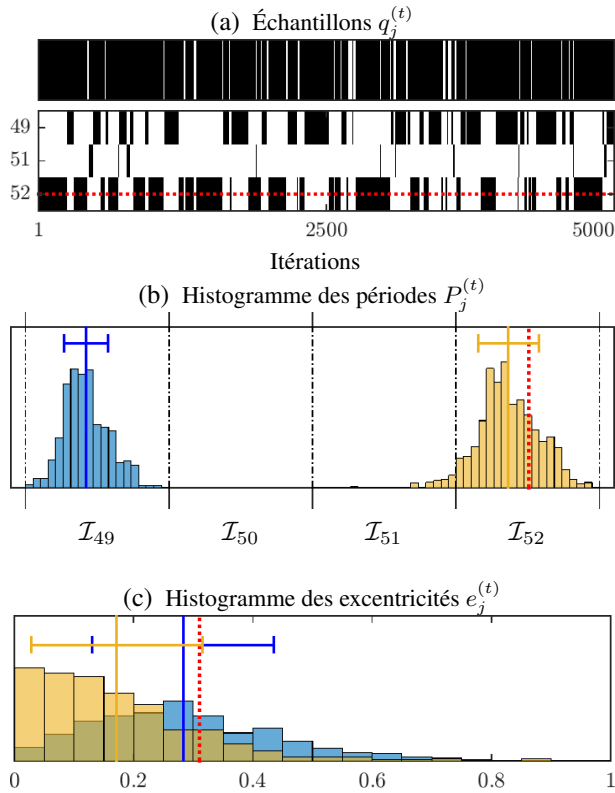
FIG. 3 – (a) Évolution de q_j^{(t)} pour j \in \Omega sur les 5000 dernières itérations (en noir q_j^{(t)} = 1 ). Au dessus, évolution de q_\Omega^{(t)} . (b) Histogrammes des périodes P_{j \in \Omega}^{(t)} , en regroupant par couleur les deux modes (bleu et jaune), dont les moyennes sont représentées par des traits verticaux avec barres d'erreur à \pm 1\sigma . Le trait rouge vertical indique la valeur théorique. (c) Histogrammes des excentricités e_{j \in \Omega}^{(t)} , où les couleurs sont relatives au mode associé.
