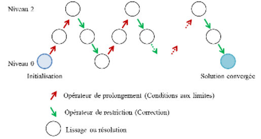
FIGURE 2 – Processus itératif de la méthode multi-grilles Local Defect Correction
