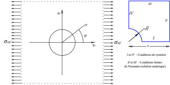
FIGURE 3 – Cas test : plaque infinie avec un trou circulaire / domaine de calcul et conditions aux limites
