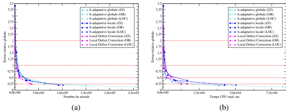
FIGURE 7 – Plaque trouée / raffinement à ratio ajusté : (a) Erreur relative globale en fonction de nombre de noeuds N_{tot} ; (b) Erreur relative globale en fonction de temps CPU total
