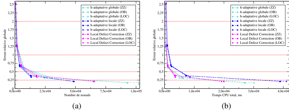
FIGURE 6 – Plaque trouée / raffinement à ratio fixe : (a) Erreur relative globale en fonction de nombre de noeuds N_{tot} ; (b) Erreur relative globale en fonction de temps CPU total
