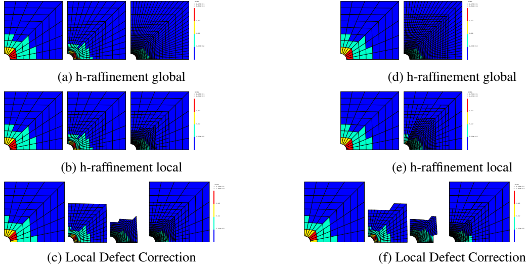
FIGURE 5 – Plaque trouée / cartes d’erreur locale réelle relative / critère d’optimalité de maillage ZZ / tolérance sur l’erreur 2 \cdot 10^{-2} / (a), (b), (c) raffinement à ratio fixe ; (d), (e), (f) raffinement à ratio ajusté.
