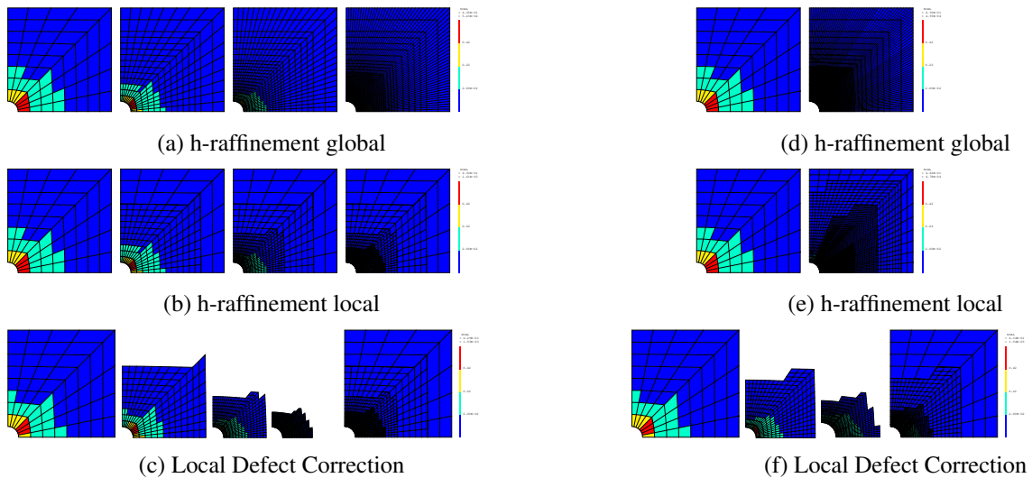
FIGURE 4 – Plaque trouée / cartes d'erreur locale réelle relative / critère d'optimalité de maillage LOC / tolérance sur l'erreur 2 \cdot 10^{-2} / (a), (b), (c) raffinement à ratio fixe ; (d), (e), (f) raffinement à ratio ajusté.
