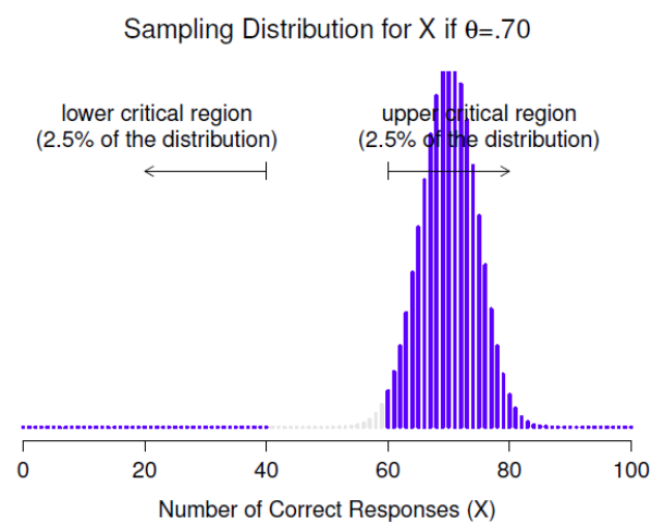
Figure 9-6 : Distribution de l'échantillonnage sous l'hypothèse alternative pour une valeur de paramètre de population de \theta = .70 . Presque toute la distribution se trouve dans la région de rejet.
