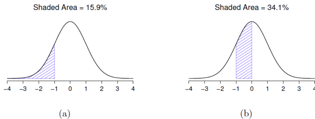
Figure 7-9 : Deux autres exemples de « l'aire sous l'idée de courbe ». Il y a 15,9 % de chances qu'une observation se situe un écart-type inférieur ou inférieur à la moyenne (panel a), et 34,1 % de chances que l'observation se situe quelque part entre un écart-type inférieur à la moyenne et la moyenne (panel b). Notez que si vous additionnez ces deux chiffres, vous obtenez 15,9\% + 34,1\% = 50\% . Pour les données normalement distribuées, il y a 50 % de chances qu'une observation soit inférieure à la moyenne. Et bien sûr, cela implique aussi qu'il y a 50 % de chances qu'elle soit supérieure à la moyenne.
