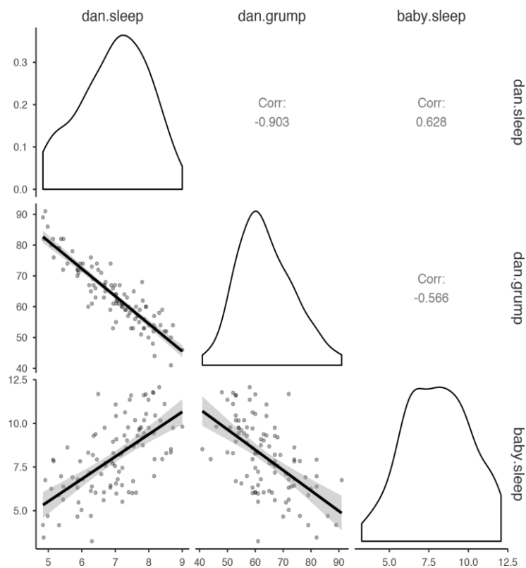
Figure 12-10 : Une matrice de nuages de points réalisé à l'aide de Jamovi.
