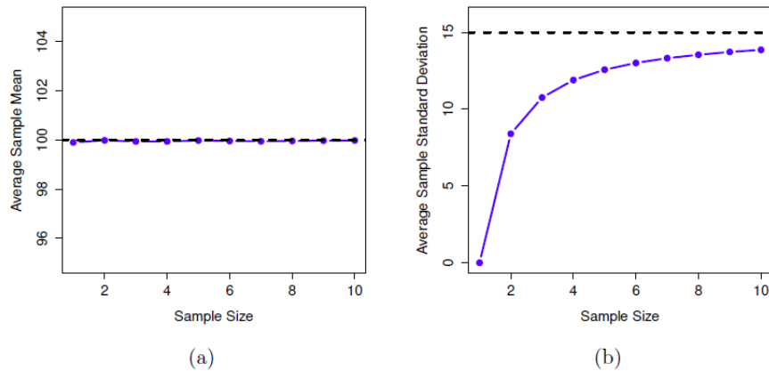
Figure 8-11 : Illustration du fait que la moyenne de l'échantillon est un estimateur non biaisé de la moyenne de la population (panel a), mais que l'écart-type de l'échantillon est biaisé (panel b). Pour la figure, j'ai généré 10 000 ensembles de données simulées avec 1 observation chacun, 10 000 autres avec 2 observations, et ainsi de suite jusqu'à une taille d'échantillon de 10. Chaque ensemble de données était constitué de fausses données sur le QI, c'est-à-dire que les données étaient normalement distribuées avec une moyenne de population réelle de 100 et un écart type de 15. En moyenne, la moyenne de l'échantillon est de 100, quelle que soit la taille de l'échantillon (panel a). Cependant, les écarts-types des échantillons s'avèrent systématiquement trop faibles (panel b), en particulier pour les petites tailles d'échantillons.
