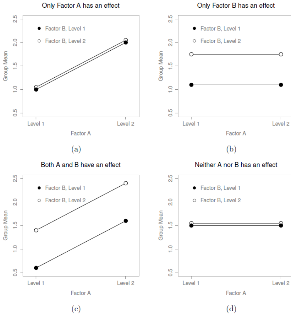
Figure 14-4 : Les quatre résultats différents d'une 2 x 2 ANOVA en l'absence d'interaction. Dans la figure (a), nous voyons un effet principal du facteur A et aucun effet du facteur B. La figure (b) montre un effet principal du facteur B mais aucun effet du facteur A. La figure (c) montre des effets principaux du facteur A et du facteur B. Enfin, la figure (d) ne montre aucun effet des deux facteurs.
