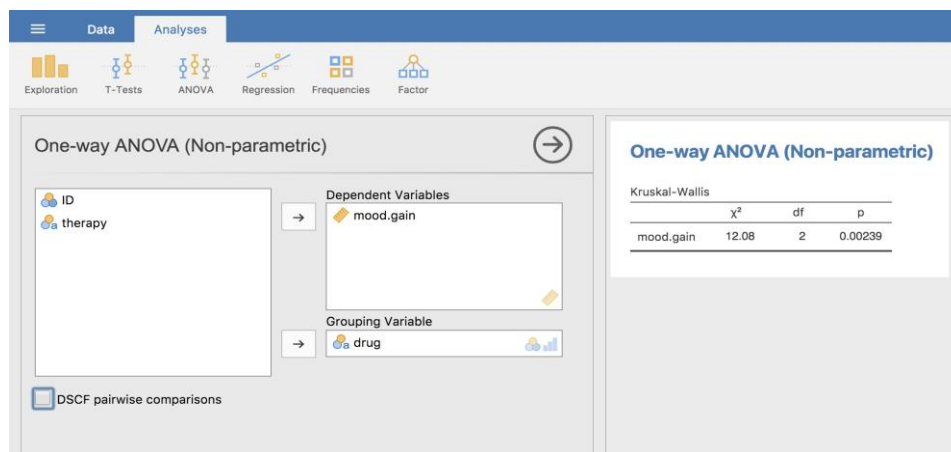
Figure 13-8 : Test non paramétrique d'ANOVA à un facteur Kruskall-Wallis avec Jamovi
