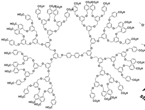
Polyether dendrimers (Fréchet et al.)
