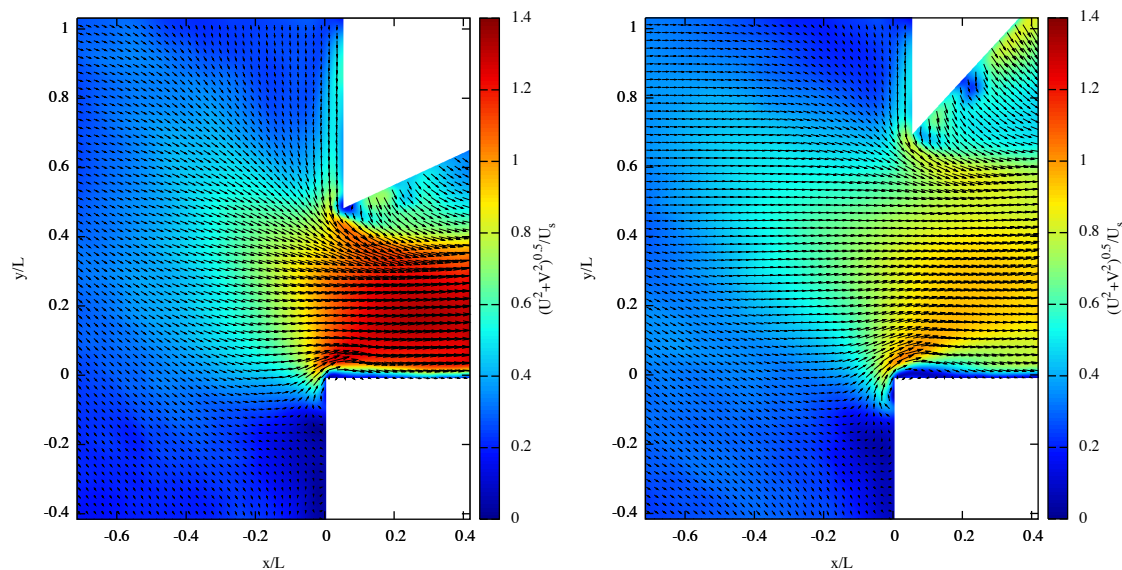
Figure 4 – Champs de vitesse moyenne pour des hauteurs d'ouverture H = 350 mm (gauche) et H = 500 mm (droite).
