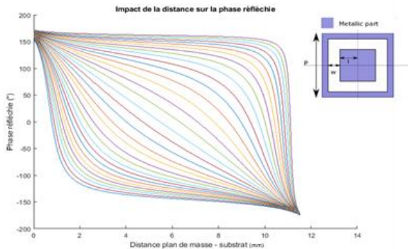
Figure 3. Phase réfléchie en fonction de h_i pour différentes géométries de cellules Phoenix.
