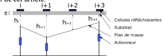
Figure 1. Schéma de principe du réseau reconfigurable proposé.
