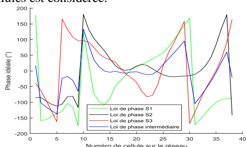
Figure 8. Nouvelles lois de phase.
