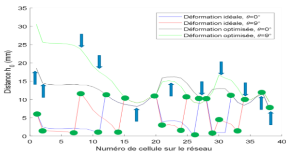
Figure 6. Distances idéales et optimales pour deux cas canoniques \theta=0^\circ et \theta=9^\circ avec un dépointage de référence sans déformation de \theta=-9^\circ .
