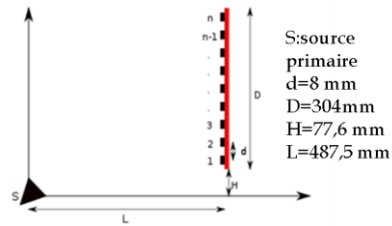
Figure 4. Géométrie de l'antenne étudiée.
