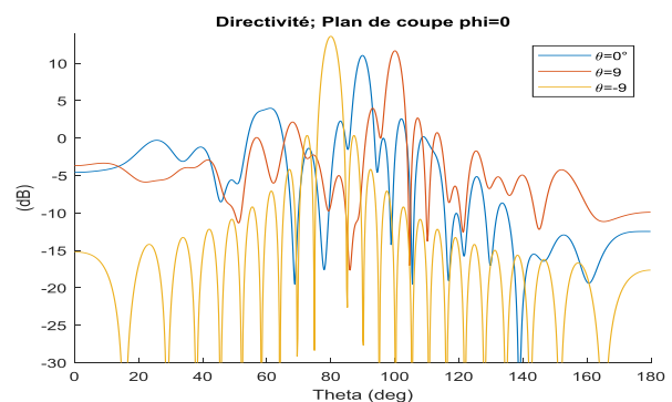
Figure 7. Comparaison des diagrammes de rayonnements obtenus pour les trois dépointages.
