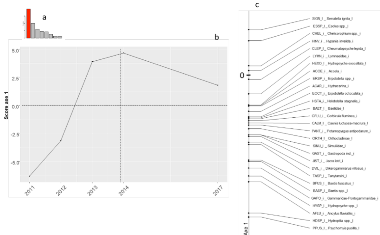
Figure 5.8 - a : graphique des valeurs propres de l'ACP; b : évolution temporelle (2011-2017) des coordonnées factorielles sur le premier axe de l'ACP des échantillonnages invertébrés; c : scores des taxons sur le premier axe de l'ACP. Afin d'améliorer la visibilité du graphique, seuls les taxons ayant un score supérieur à 0.5 sur l'axe 1 sont représentés. La ligne verticale noire signale la date de rehaussement des débits réservés.
