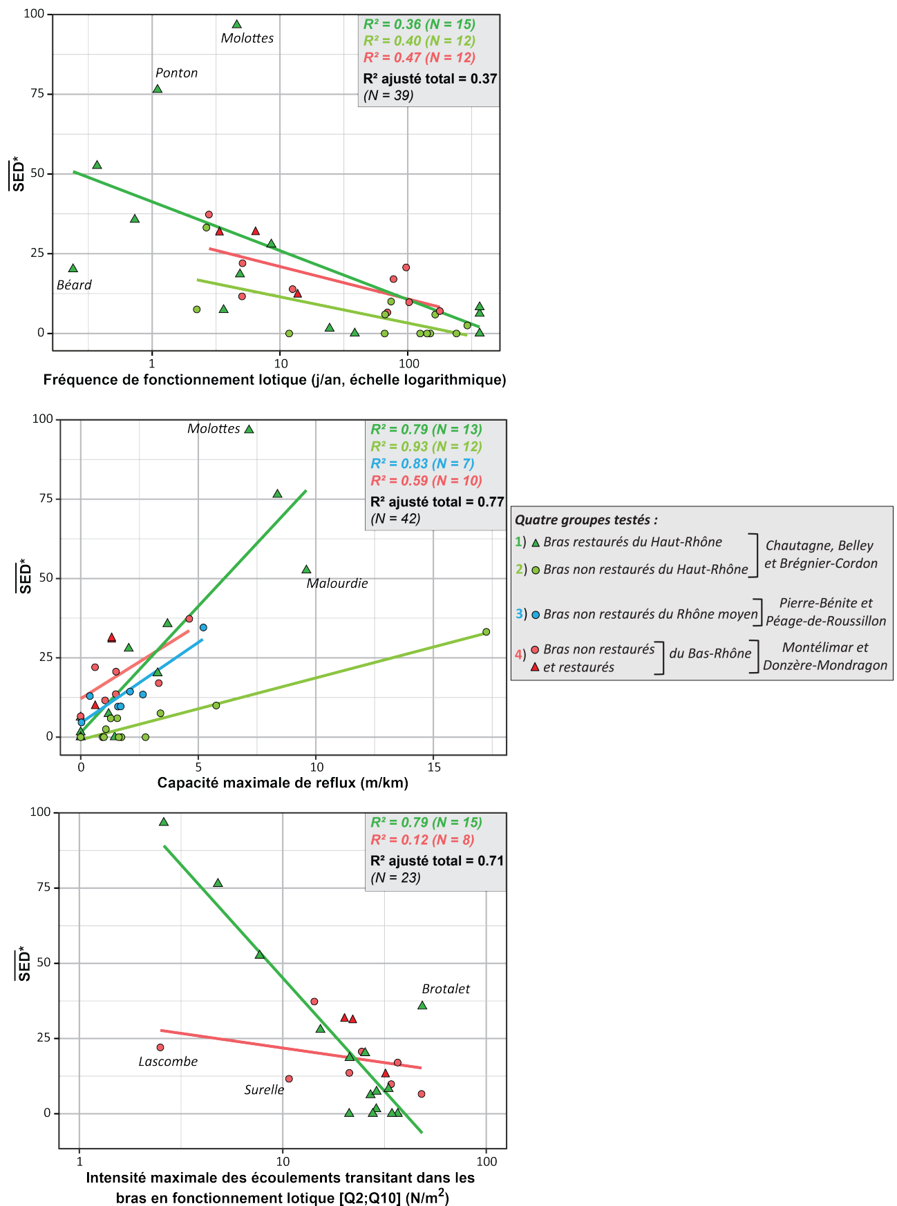
Figure 6.4 - Relations statistiques liant les vitesses de comblement normalisées et les métriques caractérisant la dynamique des écoulements de crue au sein de bras restaurés et non restaurés dans différents secteurs du Rhône (analyses de covariance). Les valeurs affichées reflètent l'état d'avancement des calculs (avril 2019).
