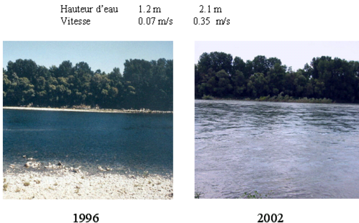
Figure 2.5 - Le vieux-Rhône de Pierre-Bénite au débit minimum avant et après augmentation
