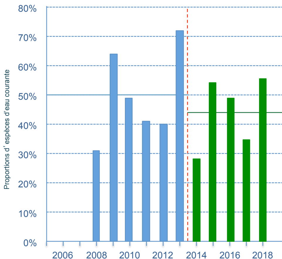
Figure 4.13 - Proportion d'espèces d'eau courante (abondances relatives des ablettes, barbeaux fluviatiles, hotus et vandoises) dans les pêches avant et après augmentation du débit réservé dans le vieux – Rhône de Montélimar. En bleu : valeurs pré-augmentation de débit minimum, en vert : valeurs post-augmentation. La ligne rouge pointillée marque la date de changement de débit réservé. La ligne continue bleue représente la valeur de la moyenne sur la période 2006-2013, la ligne verte sur la période 2014-2018.
