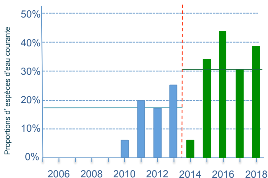
Figure 4.11 - Proportion d'espèces d'eau courante (abondances relatives des ablettes, barbeaux fluviatiles, hotus et vandoises) dans les pêches avant et après augmentation du débit réservé dans le vieux – Rhône de Baix-Le-Logis-Neuf. En bleu : valeurs pré-augmentation de débit minimum, en vert : valeurs post-augmentation. La ligne rouge pointillée marque la date de changement de débit réservé. La ligne continue bleue représente la valeur de la moyenne sur la période 2010-2013, la ligne verte sur la période 2014-2018.
