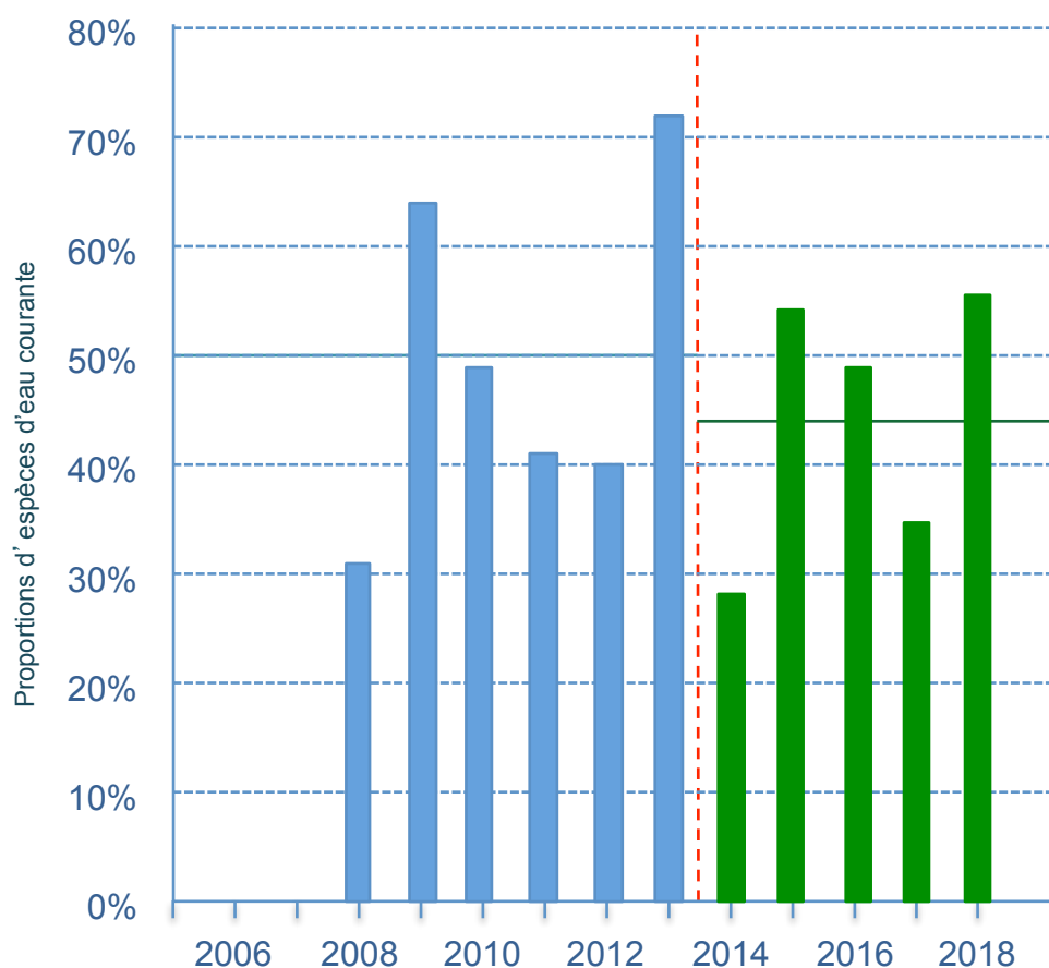
Figure 4.15 - Proportion d'espèces d'eau courante (abondances relatives des ablettes, barbeaux fluviaux, hotus et vandoises) dans les pêches avant et après augmentation du débit réservé dans le vieux – Rhône de Donzère. En bleu : valeurs pré-augmentation de débit minimum, en vert : valeurs post-augmentation. La ligne rouge pointillée marque la date de changement de débit réservé. La ligne continue bleue représente la valeur de la moyenne sur la période 2008-2013, la ligne verte sur la période 2014-2018.
