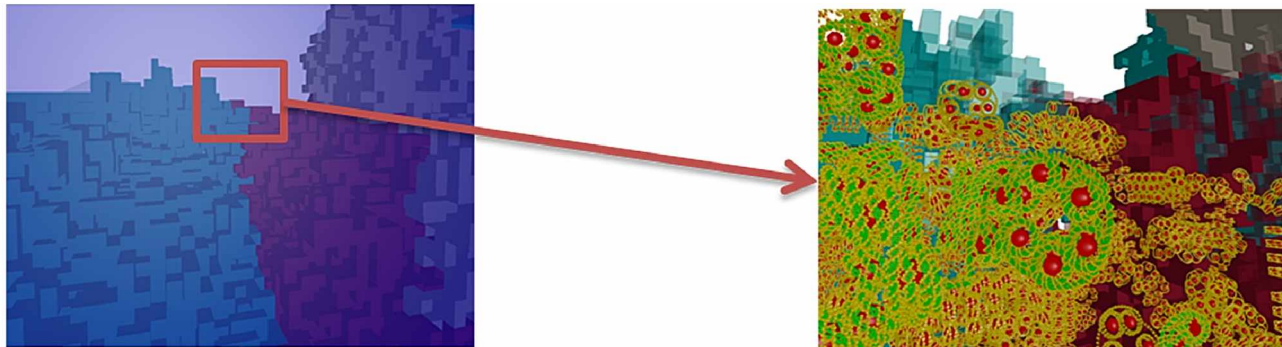
SupFig 6
