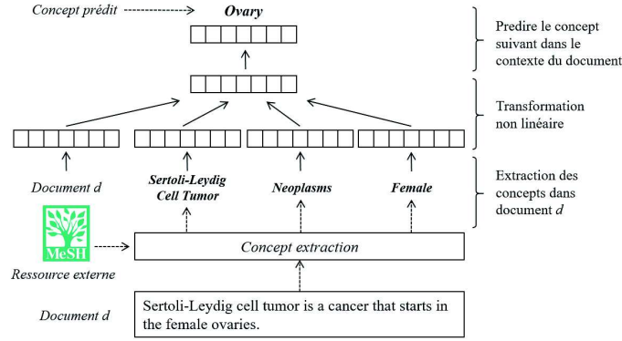
FIG. 1: Architecture du modèle conceptualDoc2vec
