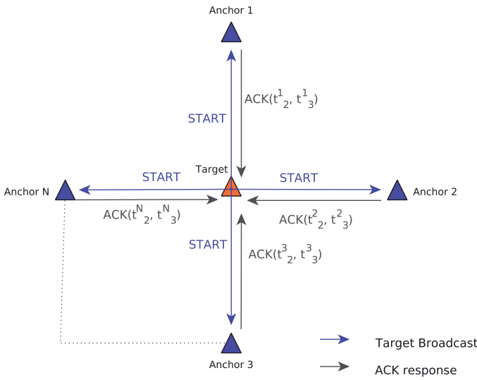
Fig. 9. The N-TWR protocol.
