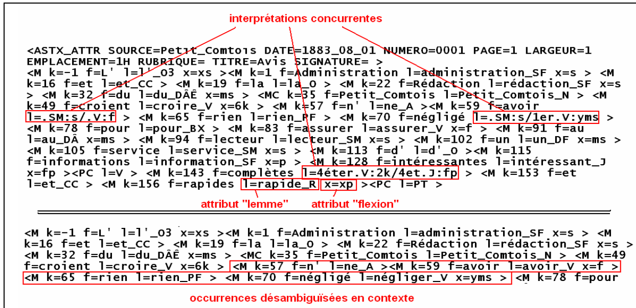
Fig. 4 : Application du dictionnaire, puis des scripts contextuels.
