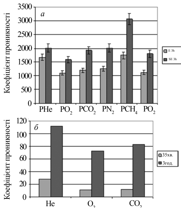
Рис. 5. Результати випробувань зразків нанопористих ПЦС мембран на газопроникність: a – поліціанурат/поліуретан (E 3h–травлення 3 години, SE-3h травлення 3 години + сенсibiлізація); б – поліціанурат/політетраметиленгліколь (травлення 35 хв. або 3 год.)
