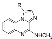
imidazo[1,2- a ]quinoxaline
