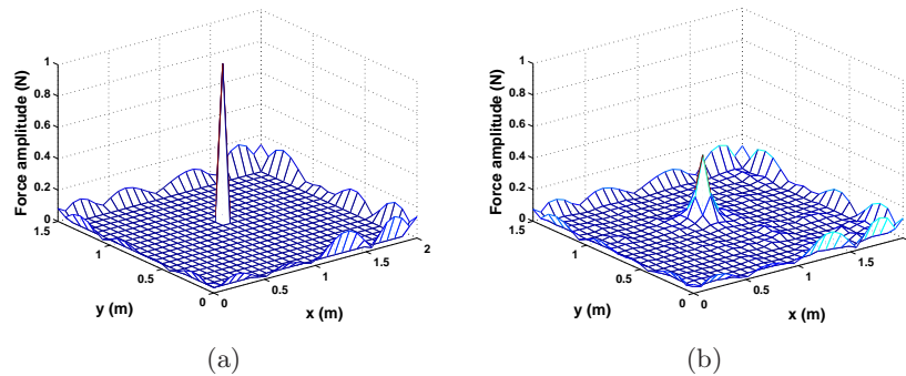
FIGURE 1 – Validation numérique - (a) Champ excitateur \mathbf{F} à identifier et (b) Champ excitateur \widehat{\mathbf{F}} identifié par la régularisation de Tikhonov
