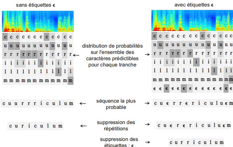
FIGURE 2 – exemple d’alignements de la fonction CTC
