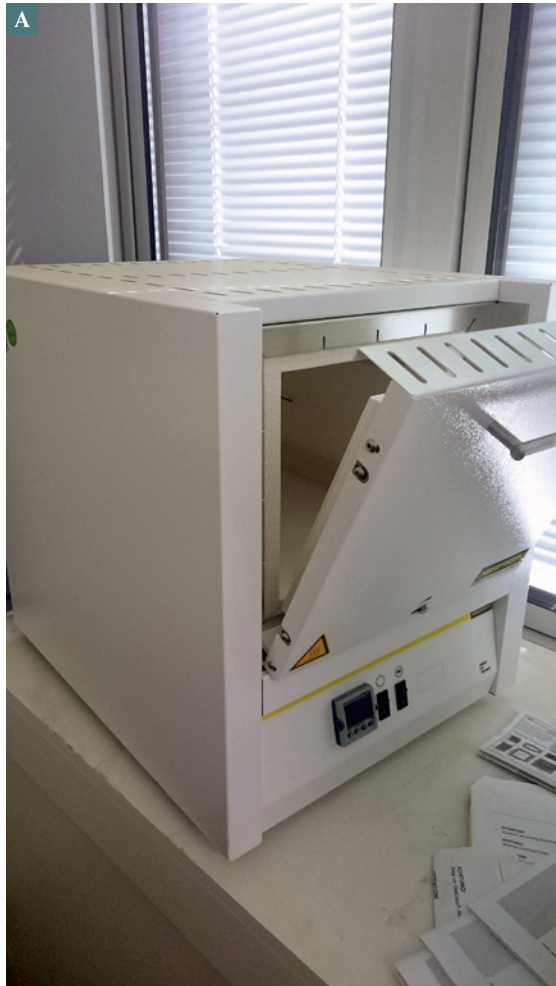
A - Le four à moufles : analyse de la matière organique présente dans chaque échantillon.
