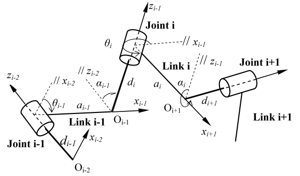
Fig. 1 Denavit–Hartenberg parameters
