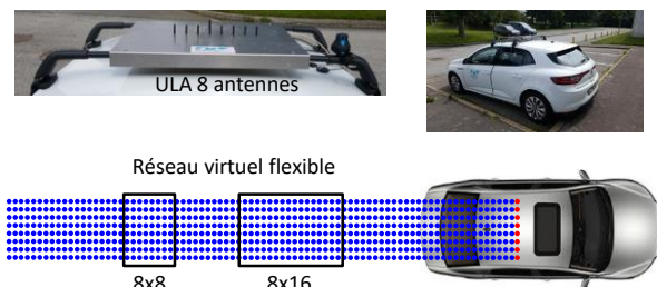
Figure 3. Principe de réseau virtuel mobile
